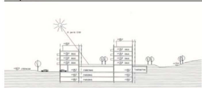
Illustrasjonssnitt vest-øst
